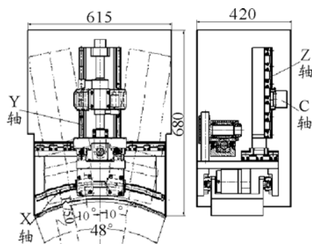
图1 透平机位移控制机构
